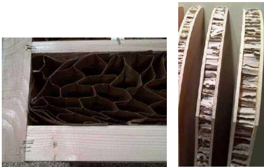
Figura 7. Pannelli compositi (tamburati)
