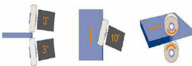
Figura 23. Regolazione dei dischi panno/fibra per garantire la migliore efficacia
